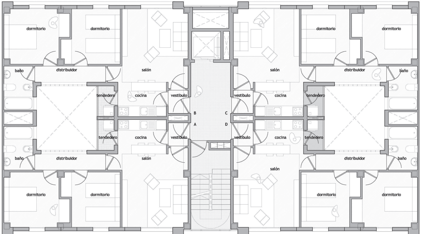
Ohiko solairu oinplanoa.
